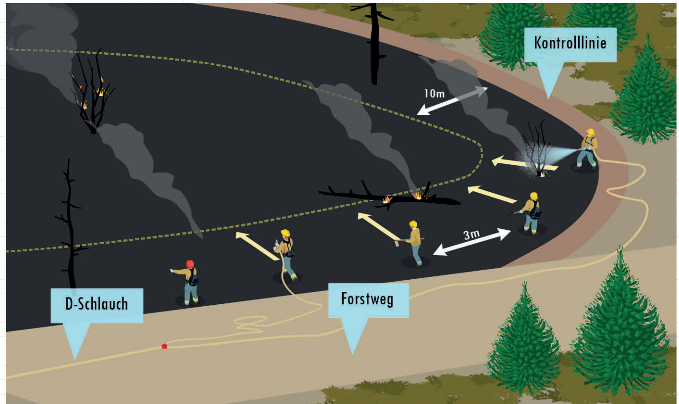
Abbildung 5. Die Zonierung und das versetzte Absuchen der Brandfläche ist wichtig. Ein guter Abstand zwischen jeder Einsatzkraft ist 3 m. Auf größeren Brandflächen empfiehlt es sich, einen bestimmten Korridor von der Feuer-/Kontrolllinie festzulegen, der abgesucht wird. Die hinter diesem Korridor gelegene Brandfläche kann ausgespart werden. Die gelbgestrichelte Linie in der Abbildung markiert die Tiefe eines solchen Korridors, der abzusuchen ist (z.B. 10 m bei dieser Brandfläche). Bei einer größeren Brandfläche würden die Einsatzkräfte in der Abbildung eine Kette von der Feuer-/Kontrolllinie bis zur vorher festgelegten Tiefe des Korridors bilden. Bei der Bemessung der Tiefe des abzusuchenden Korridors sind insbesondere die Windbedingungen einzubeziehen (mögliche Flugfeuer).
