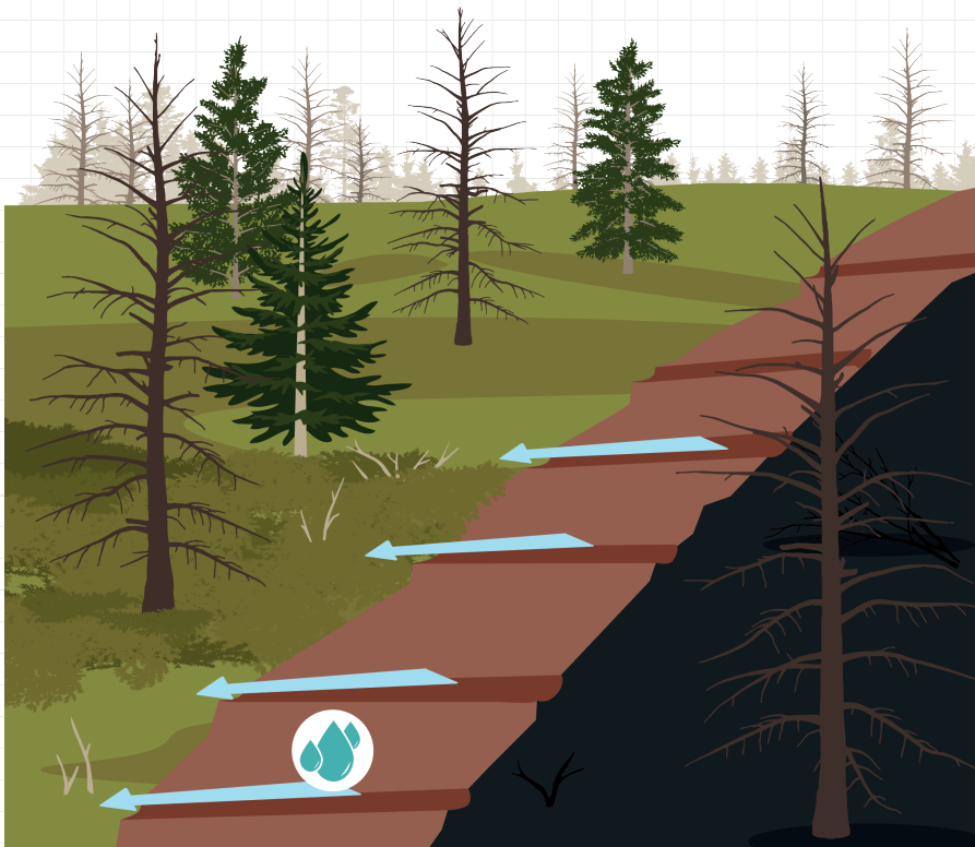
Abbildung 7. Ablaufrinnen, die diagonal über die Feuerlinie angelegt werden, können Erosionsschäden entgegenwirken.
