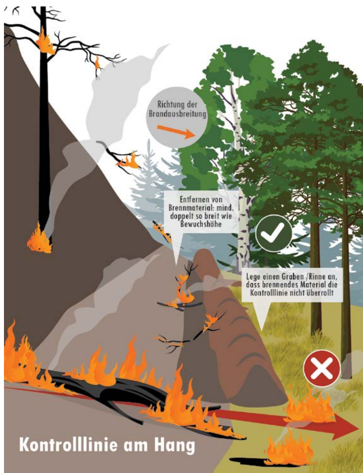
Abbildung 68 - Kontrolllinien am Hang ©EFI/WKR
