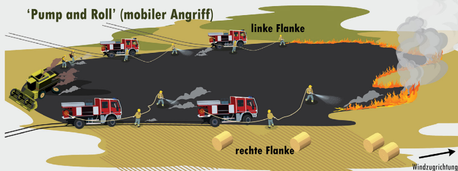
Abbildung 3.16: Pump and Roll – mobiler, fahrzeuggebundener Tandem-Angriff.
