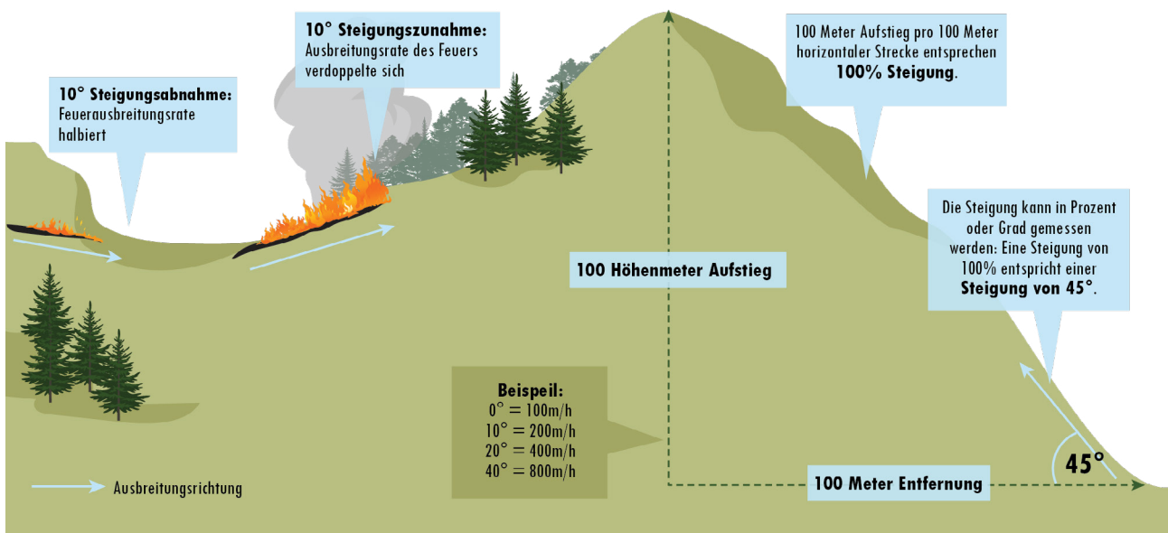
Abbildung 11 - Feuerverhalten bei Änderung der Steigung ©EFI/WKR
